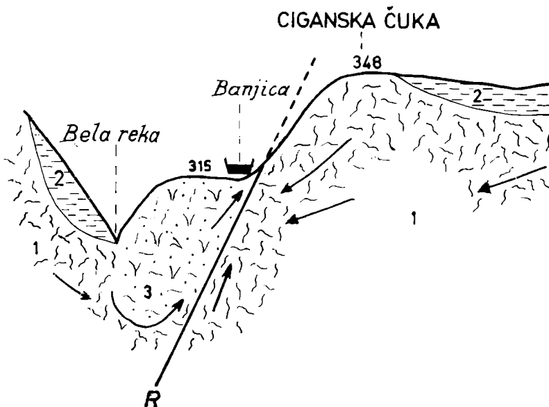
Сл. 2. — Хидрогеолошки и морфотектонски односи код Попшичне Бањице.
