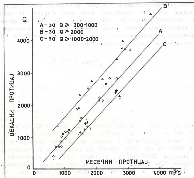
Ск. 7. -- Зависност протицаја I декаде јануара од месечног протицаја јануарског протицаја.
